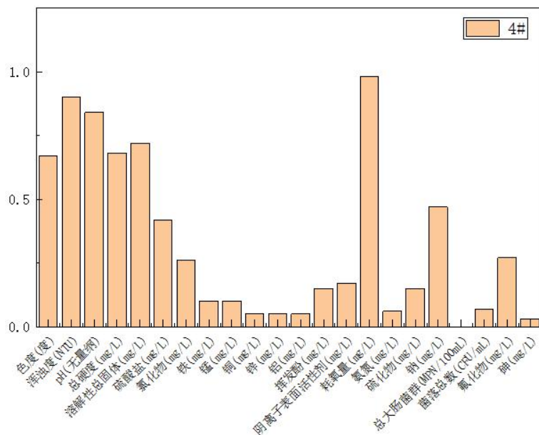
图 7.3.3-4 纳林陶亥镇截伏流饮用水水源地（4#）地下水水质评价结果
