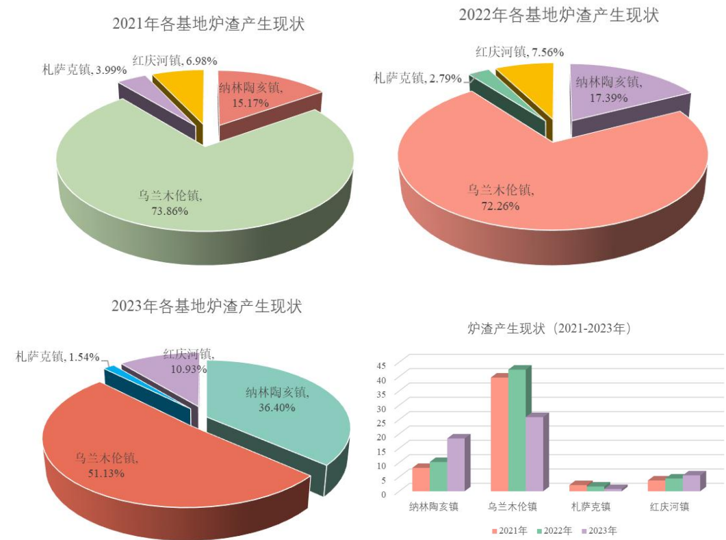
图 4.5.1-1 炉渣产生现状 (2021-2023 年)
