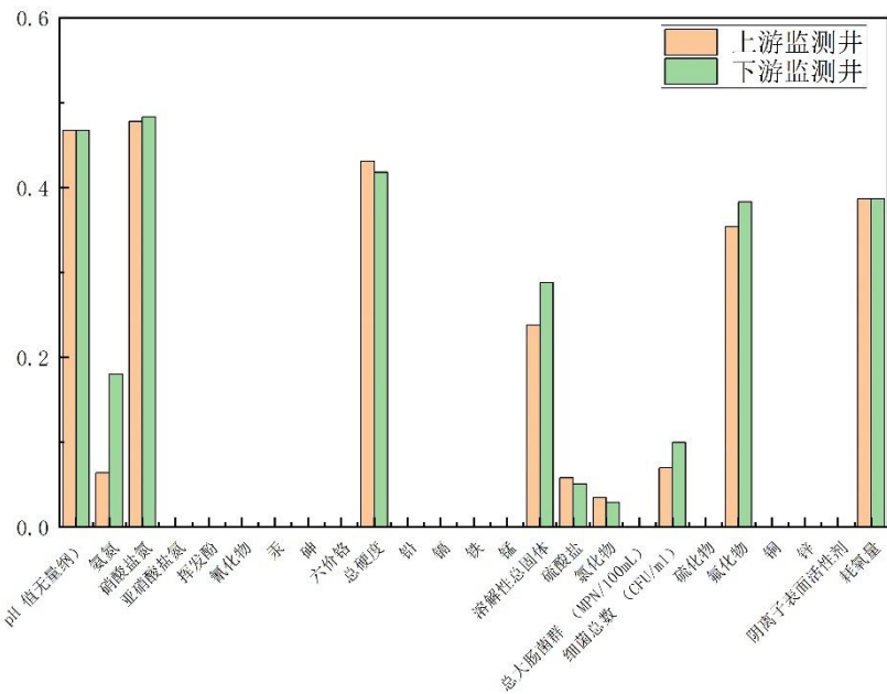
图 7.3.2-8 红庆河煤矿地下水环境质量评价结果
