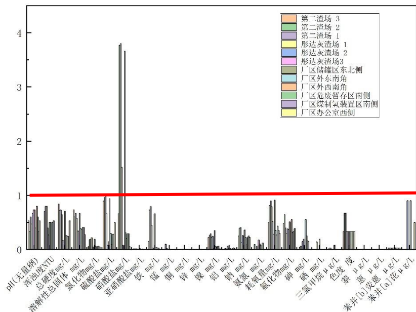
图 7.3.2-7 神华煤制油地下水水质评价结果（第二季度）
