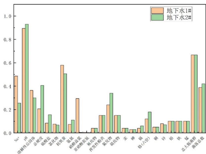
图 7.3.2-4 尔林兔煤矿地下水水质评价结果 (2022 年 5 月) (2)
