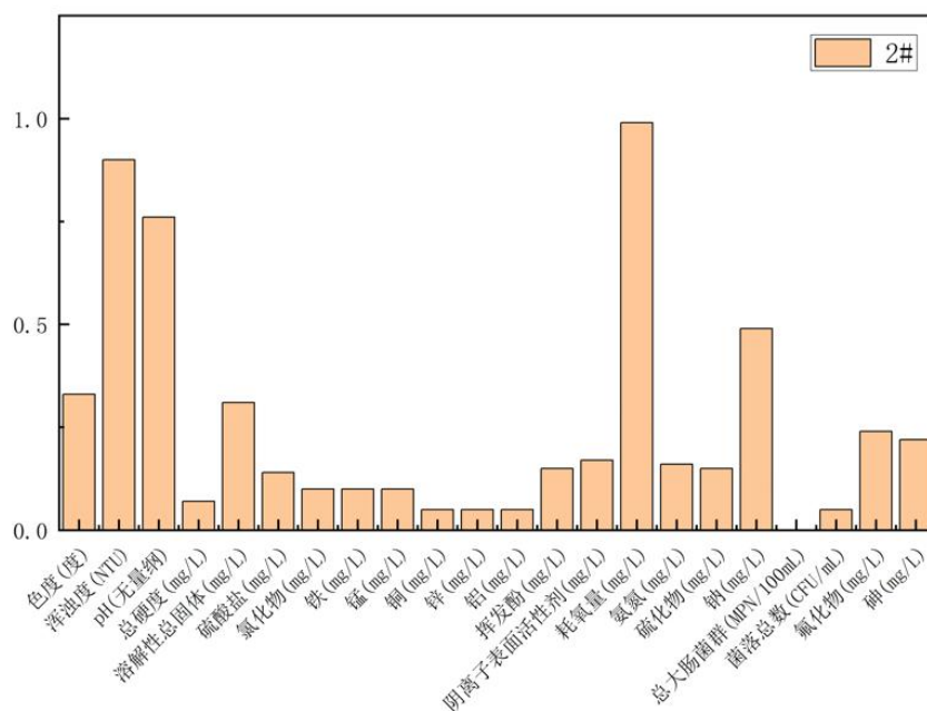
图 7.3.3-2 苏布尔嘎镇镇区水源地（2#）地下水水质评价结果
