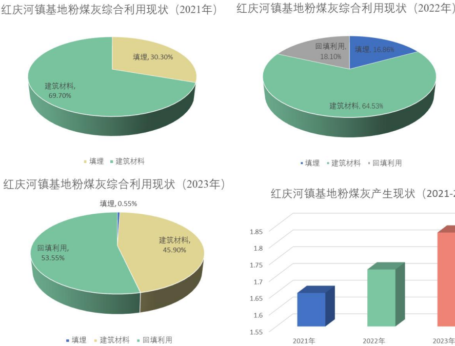
图 4.2.3-4 2021-2023 年红庆河镇基地粉煤灰综合利用现状图
