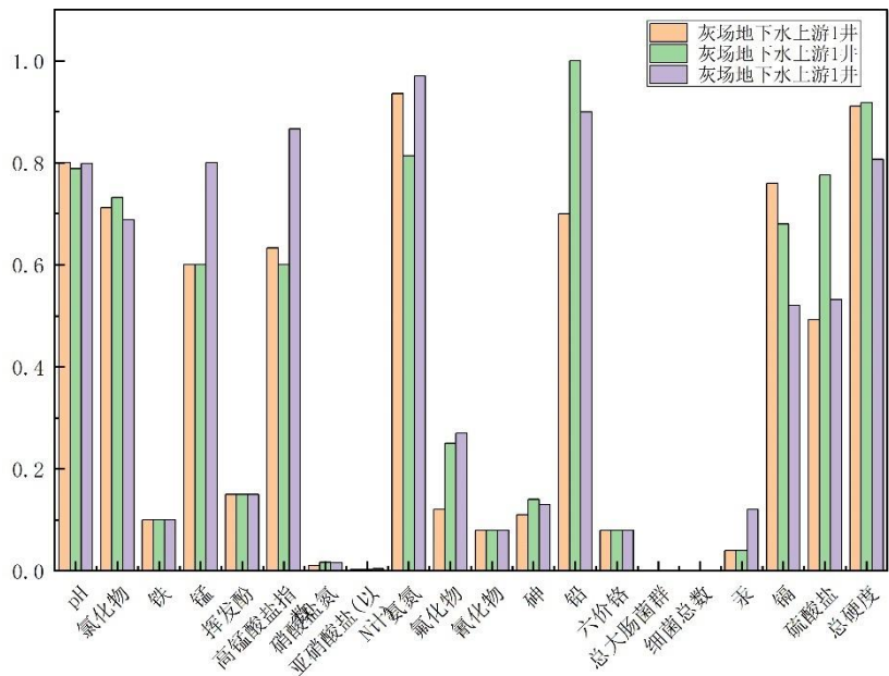
图 7.3.2-6 上湾电厂地下水水质评价结果（第一季度）（1）
