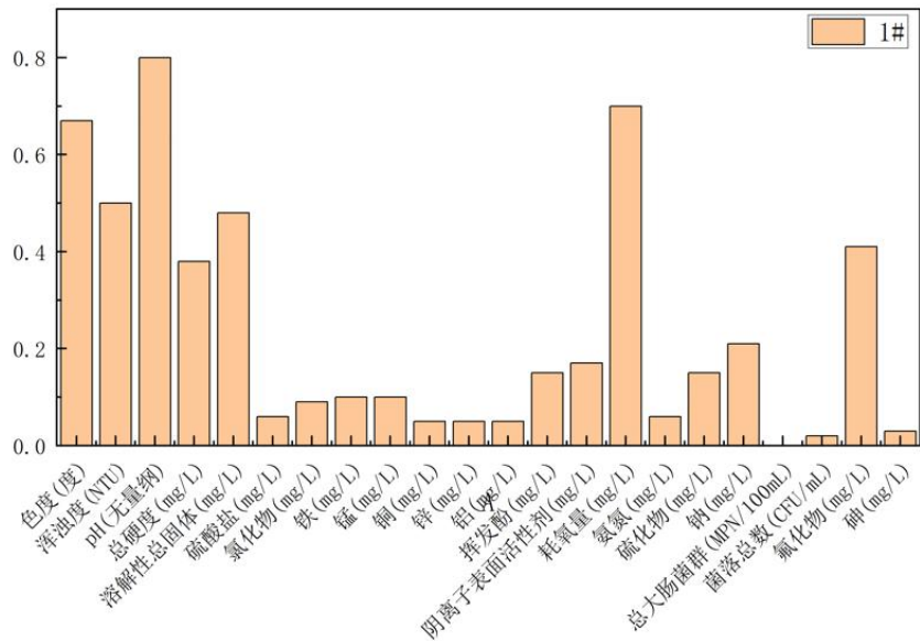
图 7.3.3-1 札萨克镇自来水水源地（1#）地下水水质评价结果
