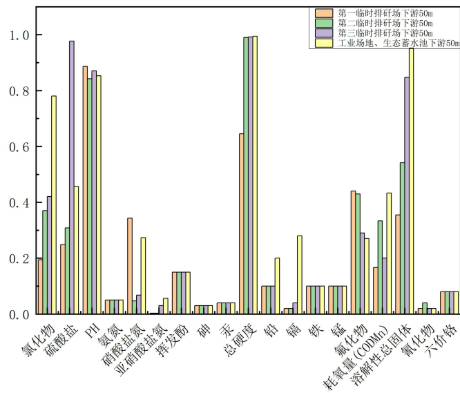
图 7.3.2-2 鑫能矿业王家塔煤矿地下水水质评价结果
