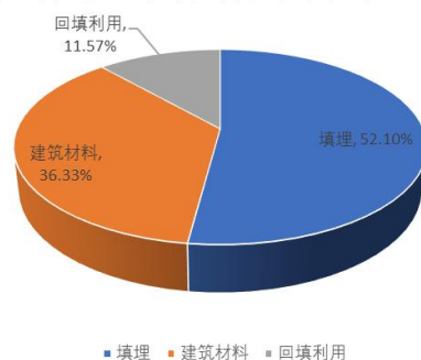
乌兰木伦镇基地粉煤灰综合利用现状（2022年）
