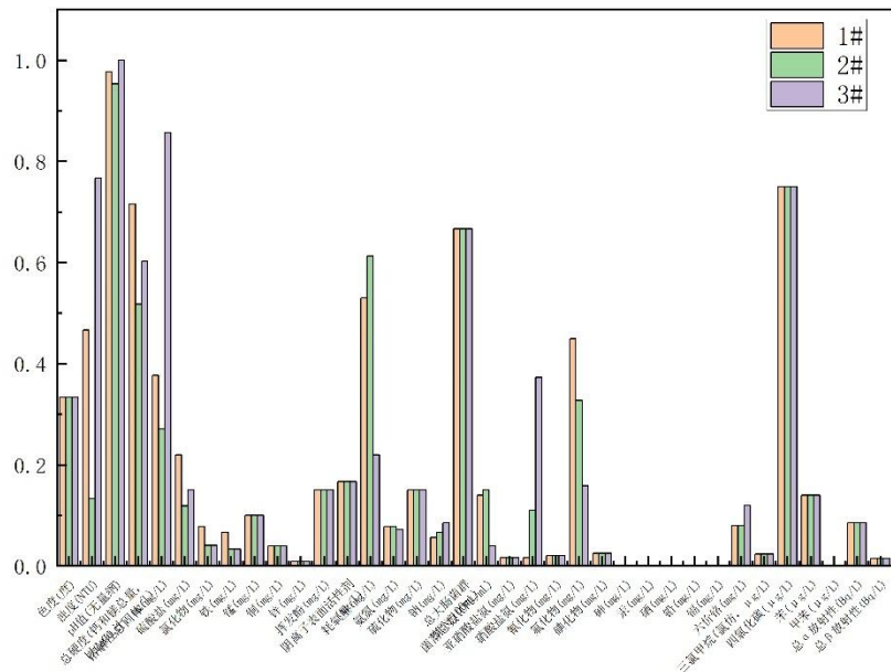
图 7.3.2-3 转龙湾煤矿地下水水质评价结果（1）
