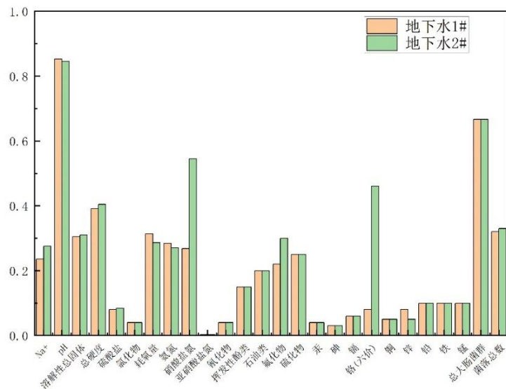
图 7.3.2-4 尔林兔煤矿地下水水质评价结果（2021 年 6 月）（1）
