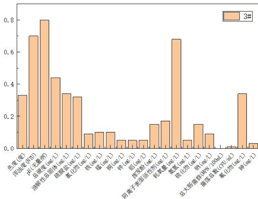
图 7.3.3-3 伊金霍洛镇水厂水源地（3#）地下水水质评价结果
