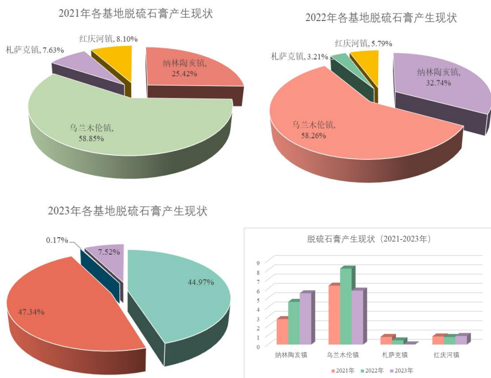
图 4.4.1-1 脱硫石膏产生现状（2021-2023 年）
