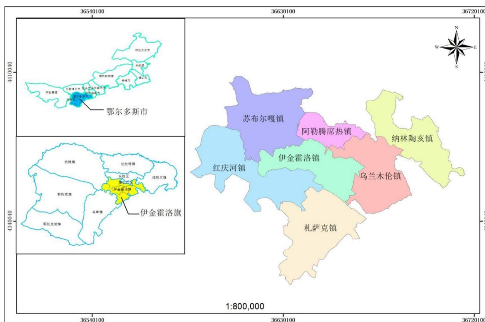
图 7.1.1-1 地理位置图
