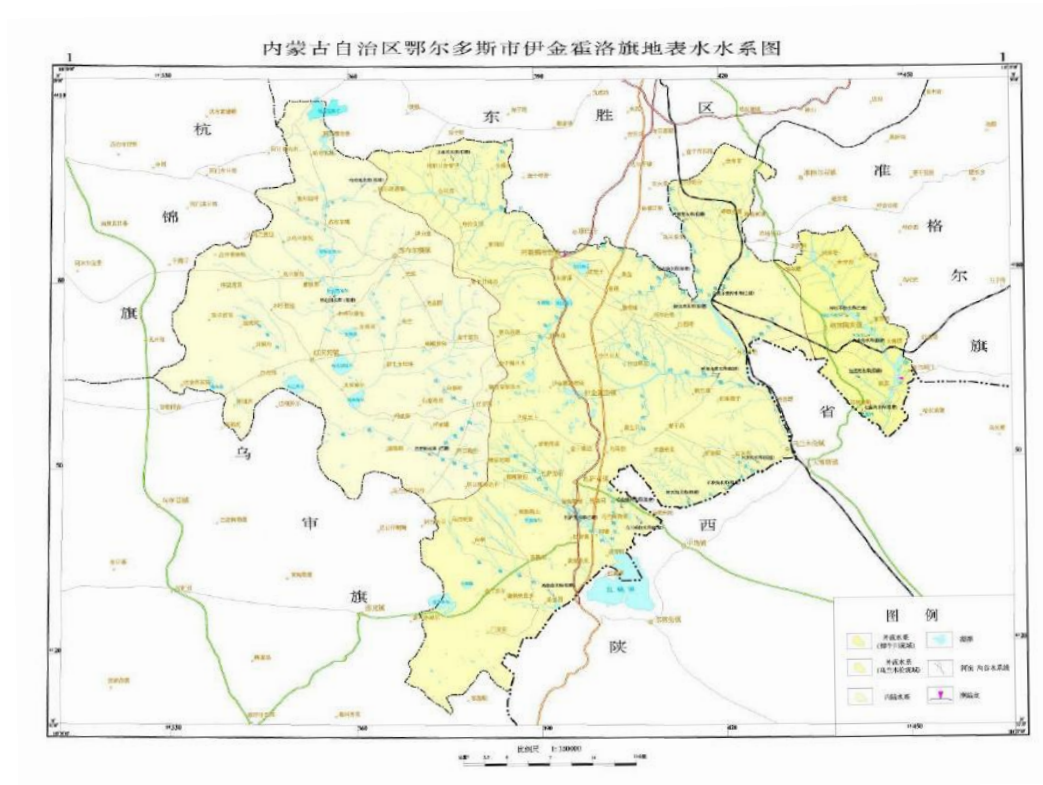
图 7.1.2-3 水系图
