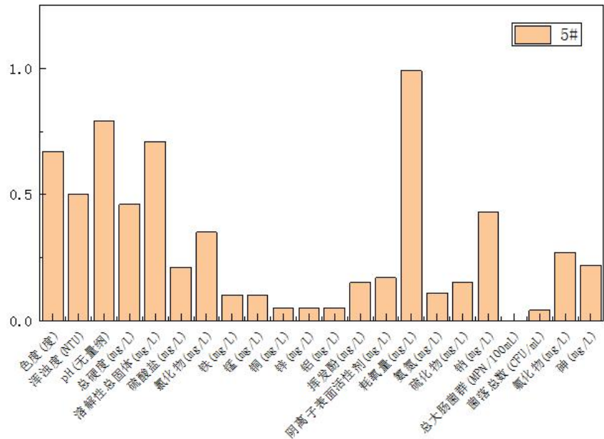
图 7.3.3-5 红庆河镇哈达图淖尔水源地（5#）地下水水质评价结果
